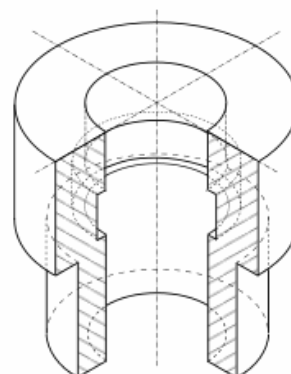
Perspective isométrique
