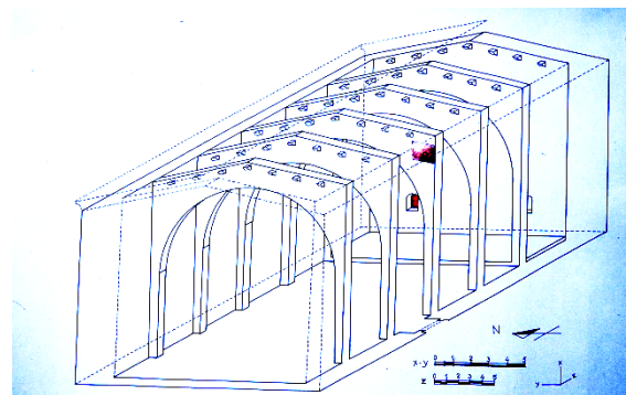
Perspectiva Caballera
